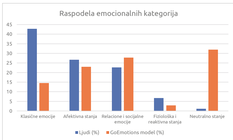
Grafikon 1. Raspodela emocionalnih kategorija u ljudskim anotacijama i predikcijama modela GouEmoušns
